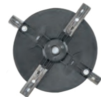
ДИСКОВИЙ НІЖ З НОЖЕМ Robolinho® 520 W Ø 20 см EAN 400 371 805 8581 Арт. № 127 466
